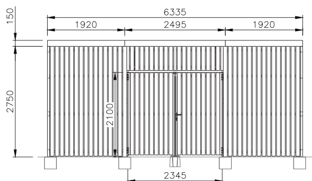
FalcoLok-600VH, 1 modul, med dobbeltdør DIN-højre og hårdtræbeklædning
